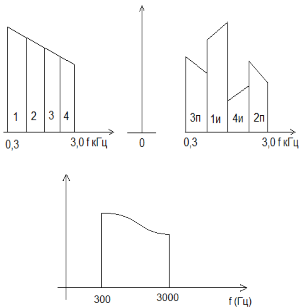
Сурет 2.6 - СЫЗЫҚТЫҚ шрамминг
