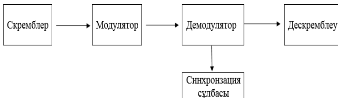
Сурет 2.1 - Сызғышты және дескремберді байланыс арнасына қосу схемасы
