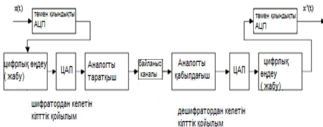
Сурет 2.2- Жиілік немесе уақытты өзгертуге негізделген қарапайым шифрлаушы сценарийлері
