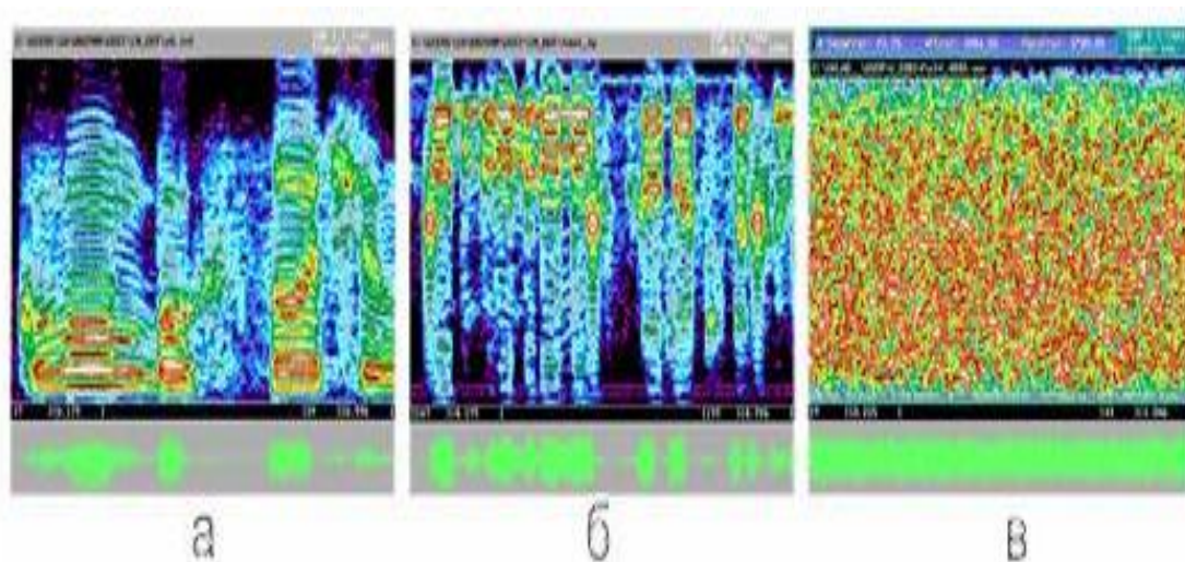
а – шығыс сөздік сигнал; б – скремблерден кейінгі сөздік сигнал; в – цифрлық түрде бергендегі сөздік сигнал (протокол V.34)
