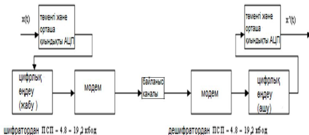
Сурет 2.3 - Сөзді жасырудағы цифрлық жүйе
